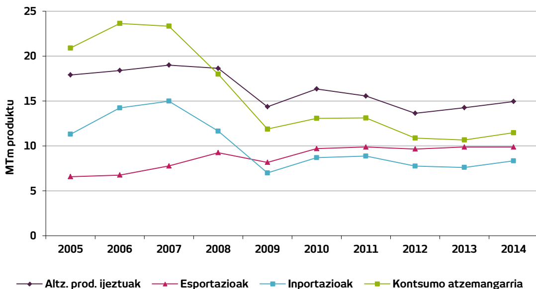
17. grafikoa Espainiako siderurgia-sektorearen magnitude nagusiak
