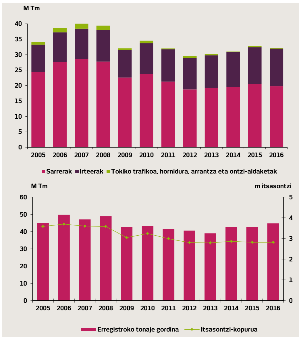
32. grafikoa Salgaien eta itsasontzien trafikoa Bilboko portuan
