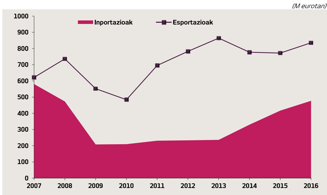
13. grafikoa Makina-tresnen sektoreko merkataritza-balantza
