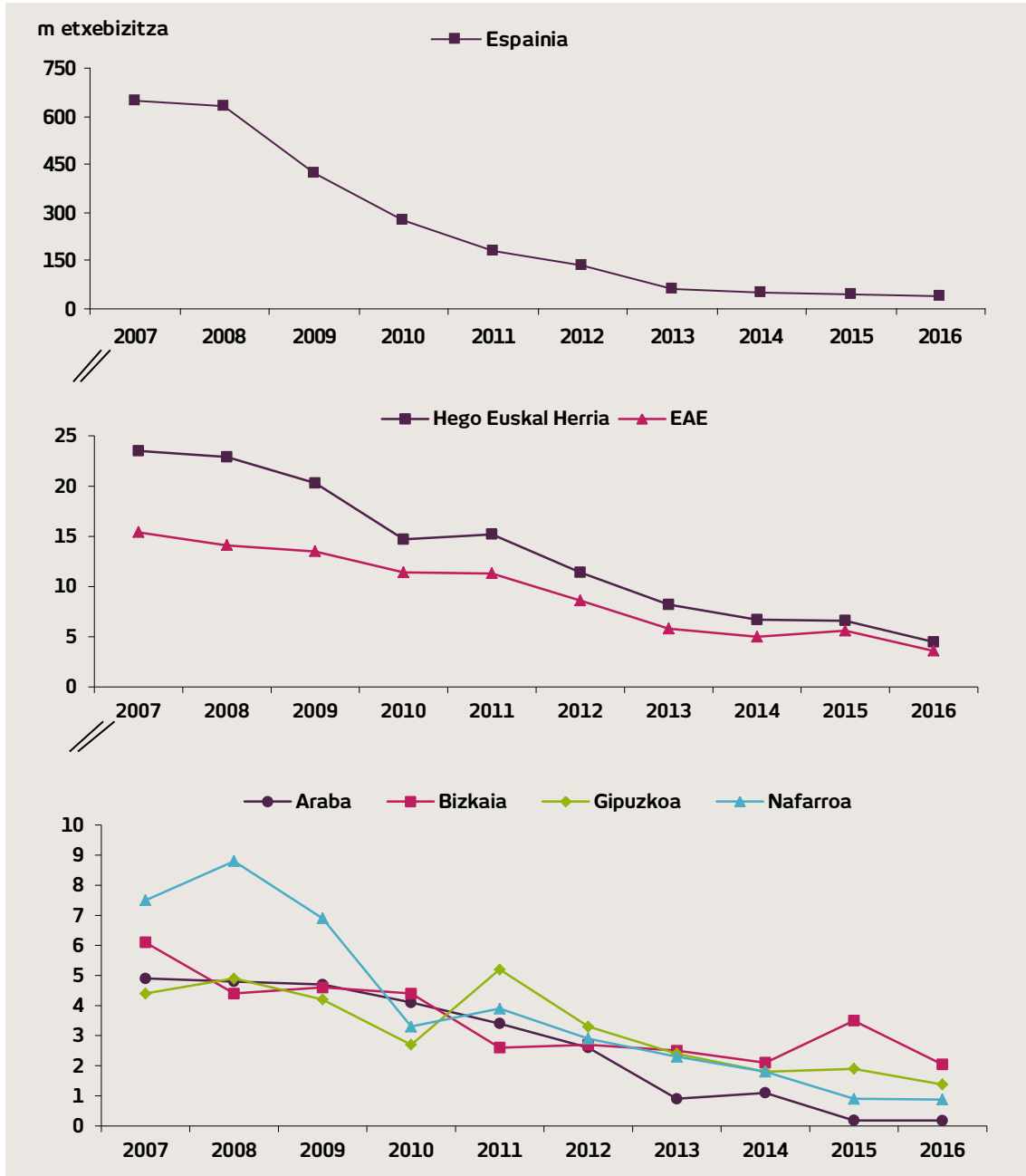
16. grafikoa Amaitutako etxebizitza-kopurua
